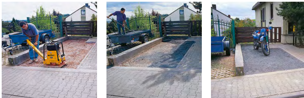
Abb. links: Verdichten der Fläche mit einem Flächenrüttler.
